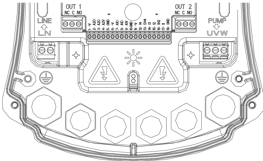
Фиг. 1: Електрически връзки
