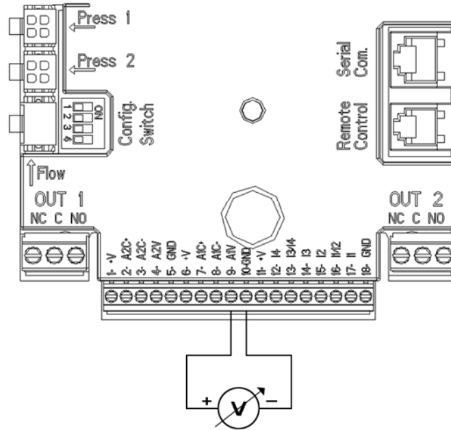
Фиг. 5: Пример на свързване на аналоговия вход
