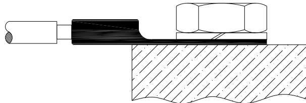
2.ábra: A védőföldelés bekötése
