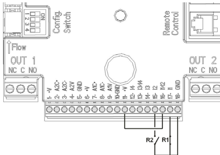
Фиг. 4: Пример за свързване на цифрови входове
