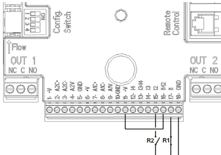
4. ábra: Példa digitális bemenetek bekötésére
